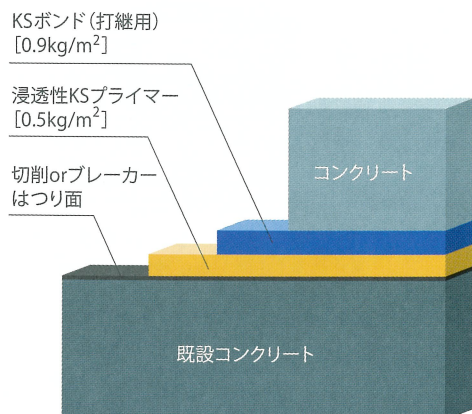
コンクリート床版 断面図
