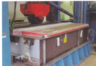
(独)土木研究所・水浸(鋼床版) 輪荷重走行試験
