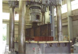
首都高速道路(株)・水浸(鋼床版) 定点疲労試験(施工技術総合研究所所有)
