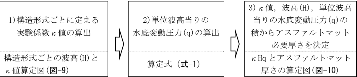
図-8 必要厚さ設計の流れ
