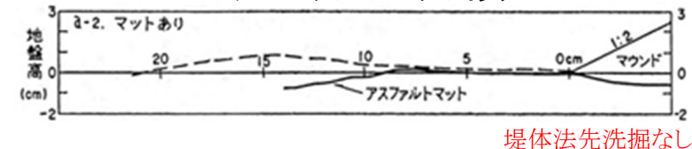
図-3 実験結果
