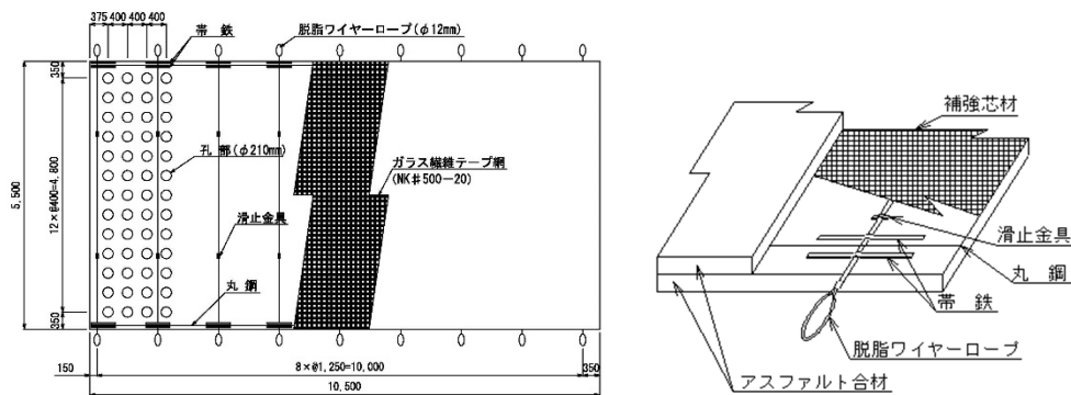
図-1 洗掘防止用アスファルトマットの構造（例）・敷設状況
