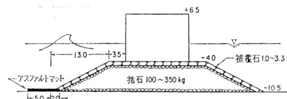
図-2 実験断面
