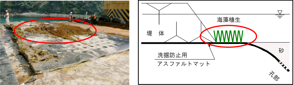
図-7 実海域でのアスファルトマットへの海藻植生(山口県・見島漁港)
