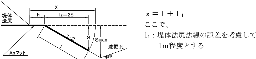
図-11 必要張出し長さの設計の流れ
