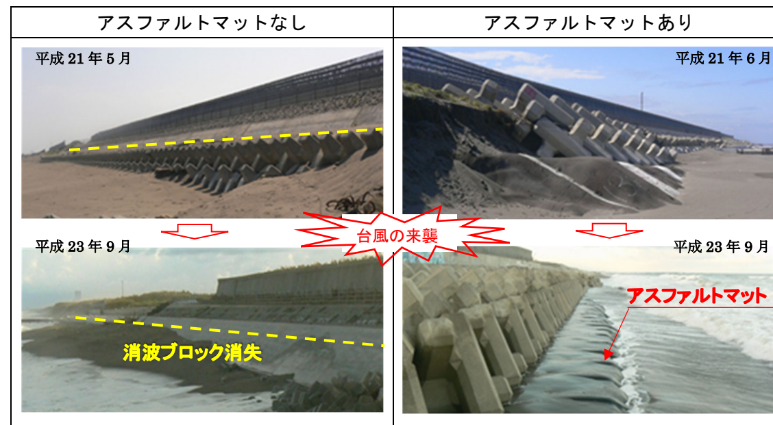
図-4 現地構造物追跡調査（アスファルトマットの効果確認）
