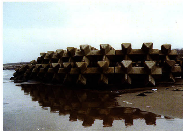
離岸堤 (昭和52年施工)
