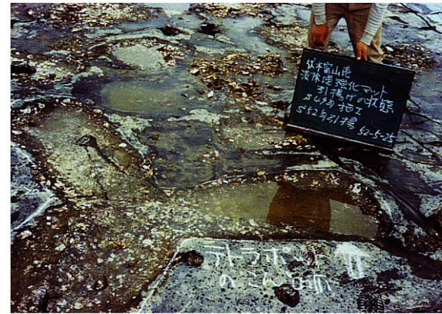
テトラポッド上載部のアスファルトマットの状況
