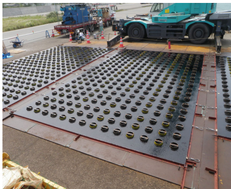
全面孔あき強化アスファルトマット製作状況
