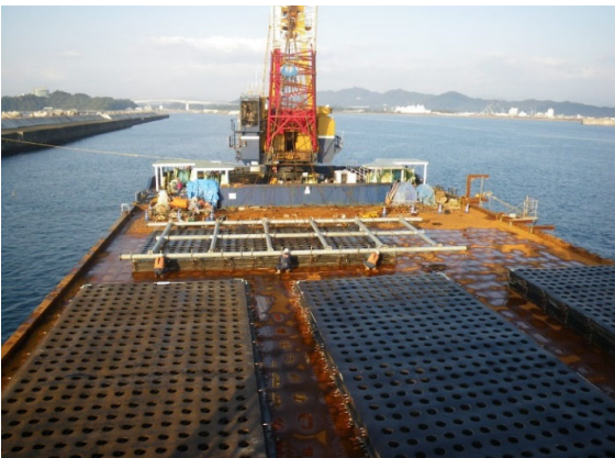
洗掘防止用全面孔あき強化アスファルトマット
