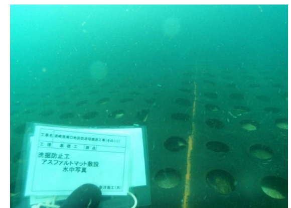
アスファルトマット敷設状況(水中)
