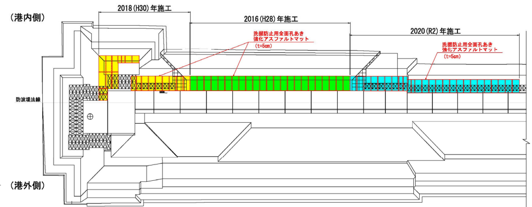
アスファルトマット敷設割付図（東防波堤）一部
