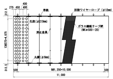
② 洗掘防止用孔あき強化アスファルトマット構造図
