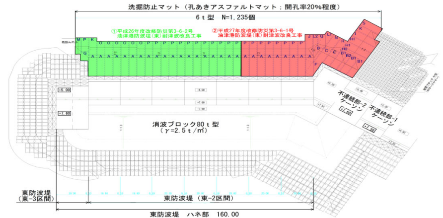
アスファルトマット敷設割付図
