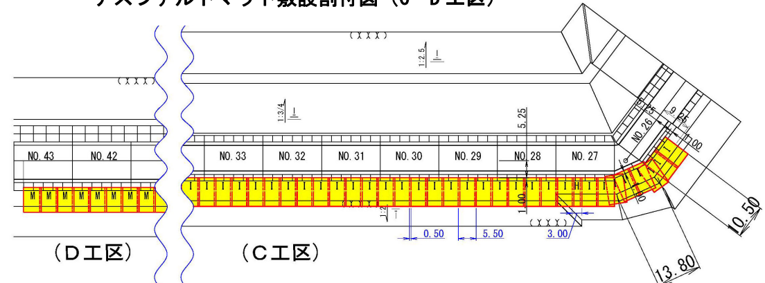
標準断面図 (C工区)
