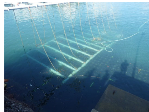
アスファルトマット敷設状況(水中)③ (スネーク吊金具使用)
