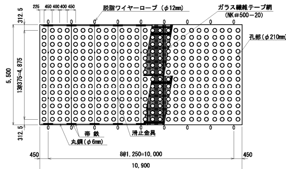
① 洗掘防止用全面孔あき強化アスファルトマット構造図
