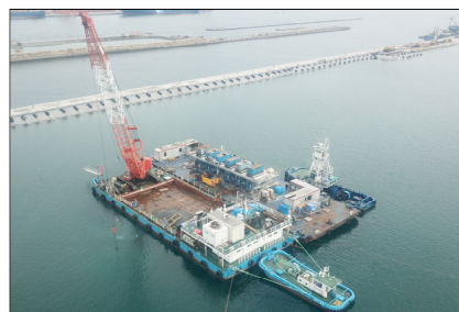
アスファルトマスチック打設状況
